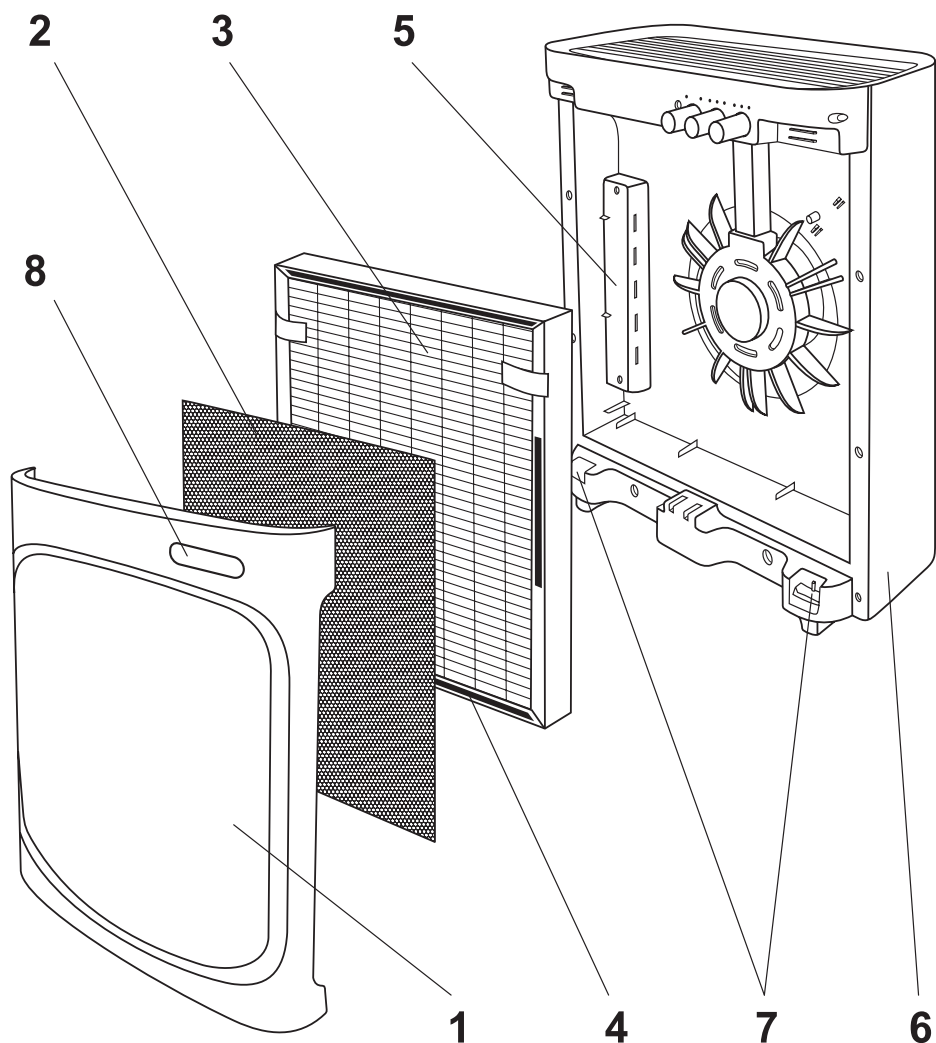
Структурная схема очистителя воздуха «АТМОС-МАКСИ-105»
